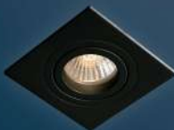
E5809BK. Aluminio. 1×GU10. 92×92mm. Orientable. Negro.
