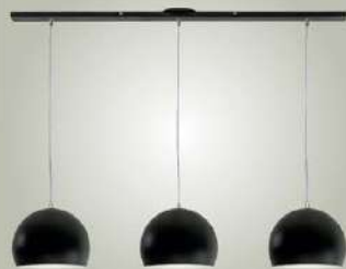
1872/C3N. 3×E27. Base 100×4cm. Negro.
