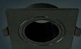
P2000N. Policarbonato. 1×GU10. 92×92mm. Orientable. Negro.
