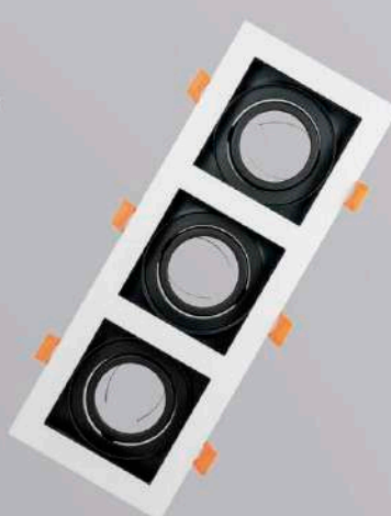
EM7003B+N. 3xGU10, 100x270mm. Metal. Orientable. Blanco + Negro.
