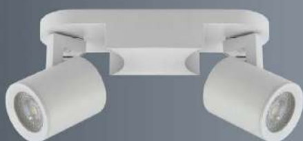
U1302B. Aluminio. 2×GU10. 22×7×12,5cm. Blanco.
