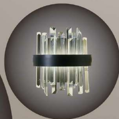
L8016. LED 16W 3000K. Ø24×25cm. Negro.
